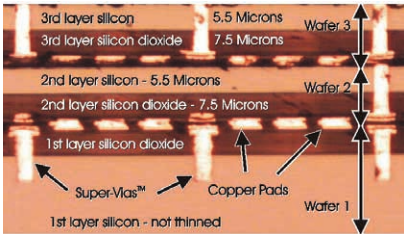
Cu-Cuの熱圧着接合 提供:Tezzaron
