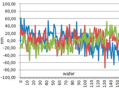
EVG SmartView® NT2 アライナーによるマラソントテストのアライメント結果。 全てのウェーハが100 nm以内の精度でアライメント
