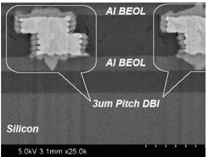
Ziptronix社による直接接合したウェーハの接合界面 提供:Ziptronix
